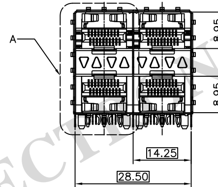
DETAIL A 1:1
