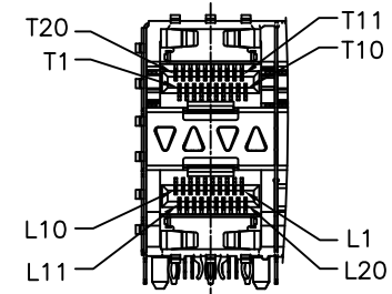
DETAIL A 1:1
