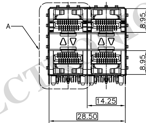
DETAIL A 1:1
